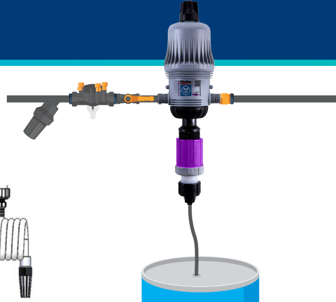
Emiş Hortumu (ağırlık ve filtrasyon sistemi ile birlikte)
